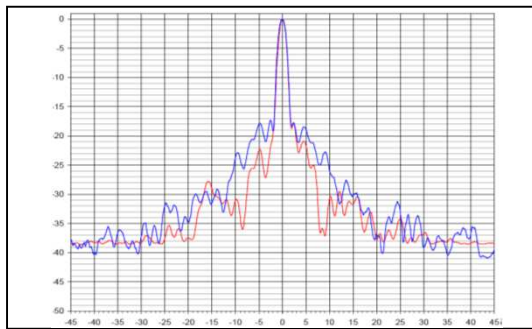
40 GHz
